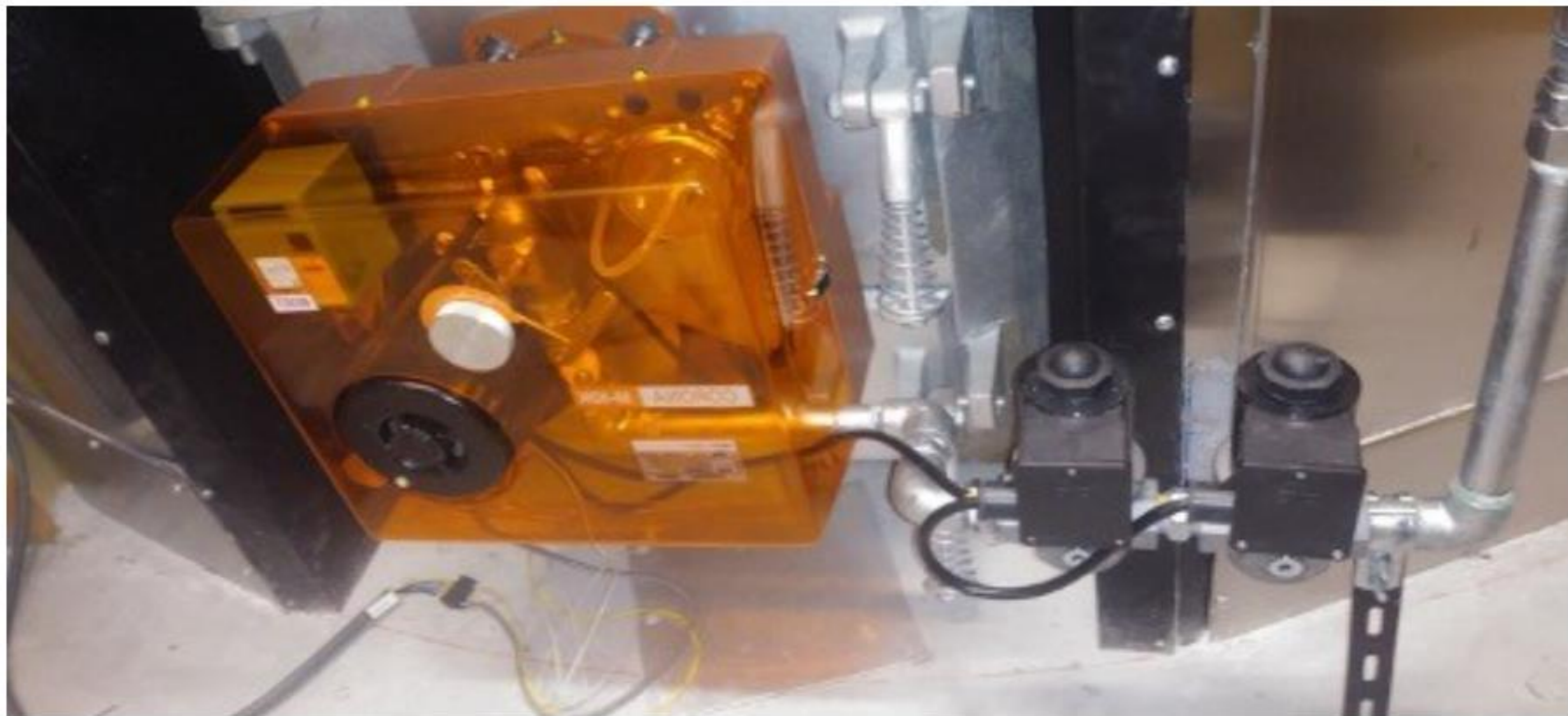
新規ガスバーナー【新設正面】ガス配管右設定 LPG仕様
